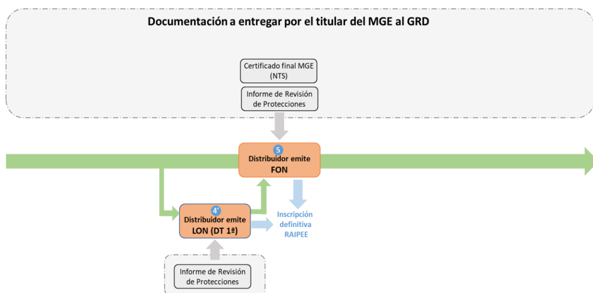
Figura 2 - Flujo de proceso de puesta en servicio de los MGE tipo A conectados a la RdD del sistema eléctrico peninsular.
