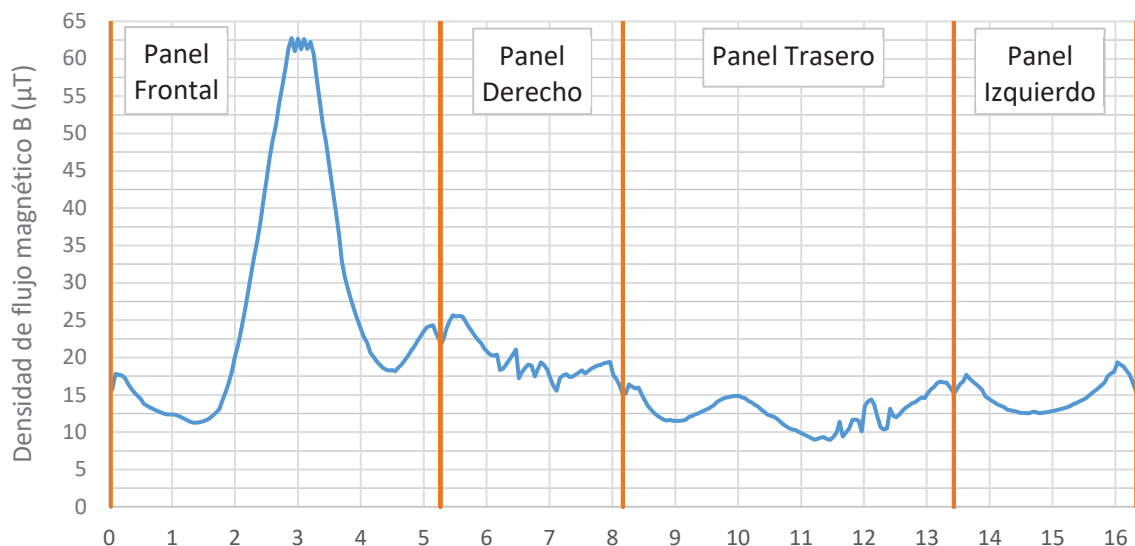
Figura 10. Densidad de flujo magnético (B[T] = Magnitud B) en envoltorio situada a 1 metro (2L+1T [Sup]).
