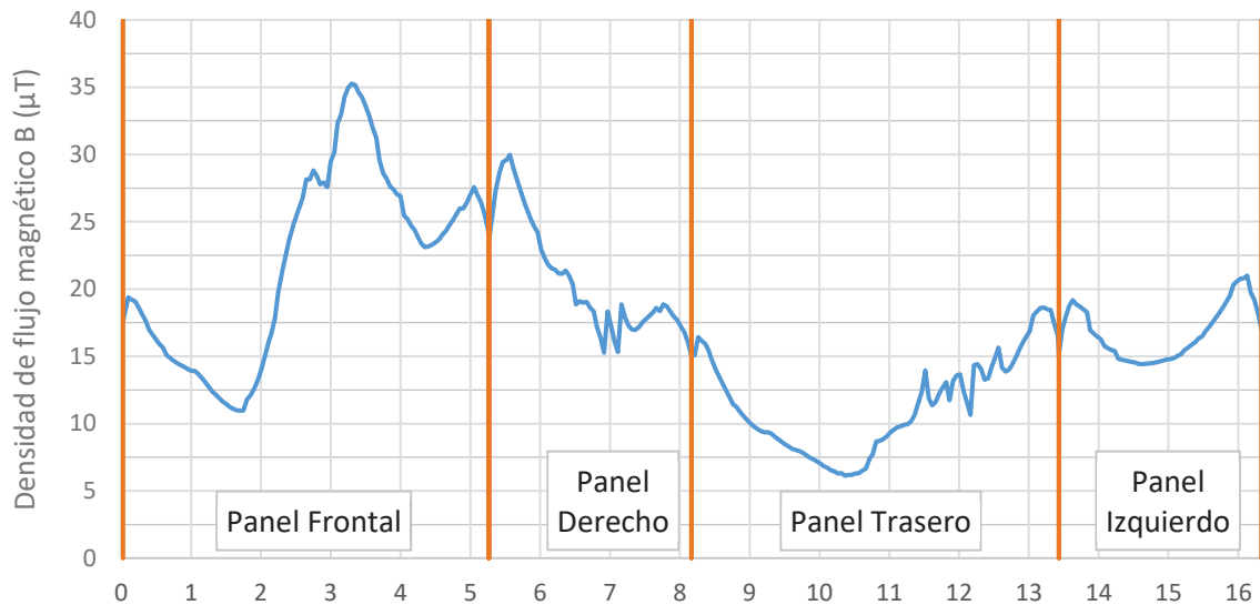
Figura 9. Densidad de flujo magnético (B[T] = Magnitud B) en envoltorio situada a 0,5 metros (2L+1T [Sup]).
