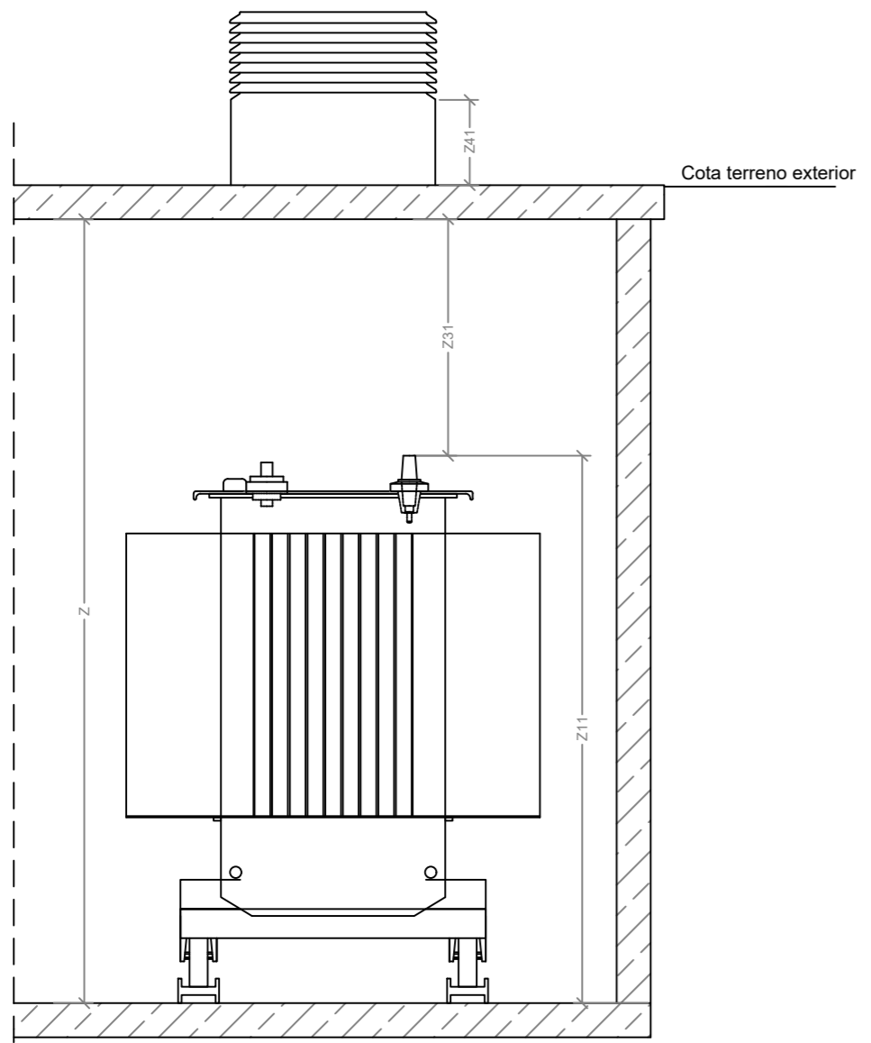
SECCION A-A'
