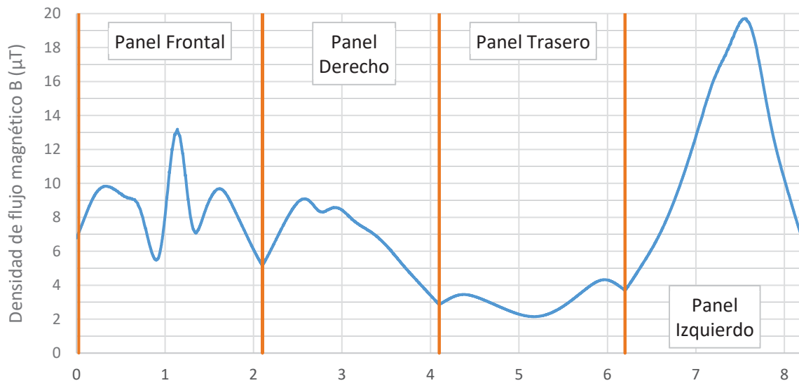
Figura 88. Densidad de flujo magnético ( B[T] = \text{Magnitud } B ) en envoltorio situada a 1 metro (3L [Semi]).
