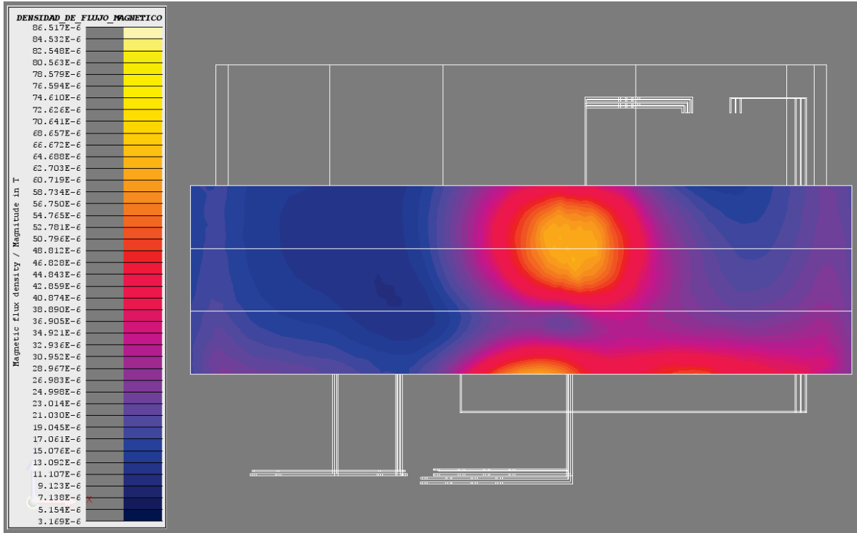
Figura 5. Densidad de flujo magnético (B[T] = Magnitud B) en el panel frontal (2L+1T [Sup]).
