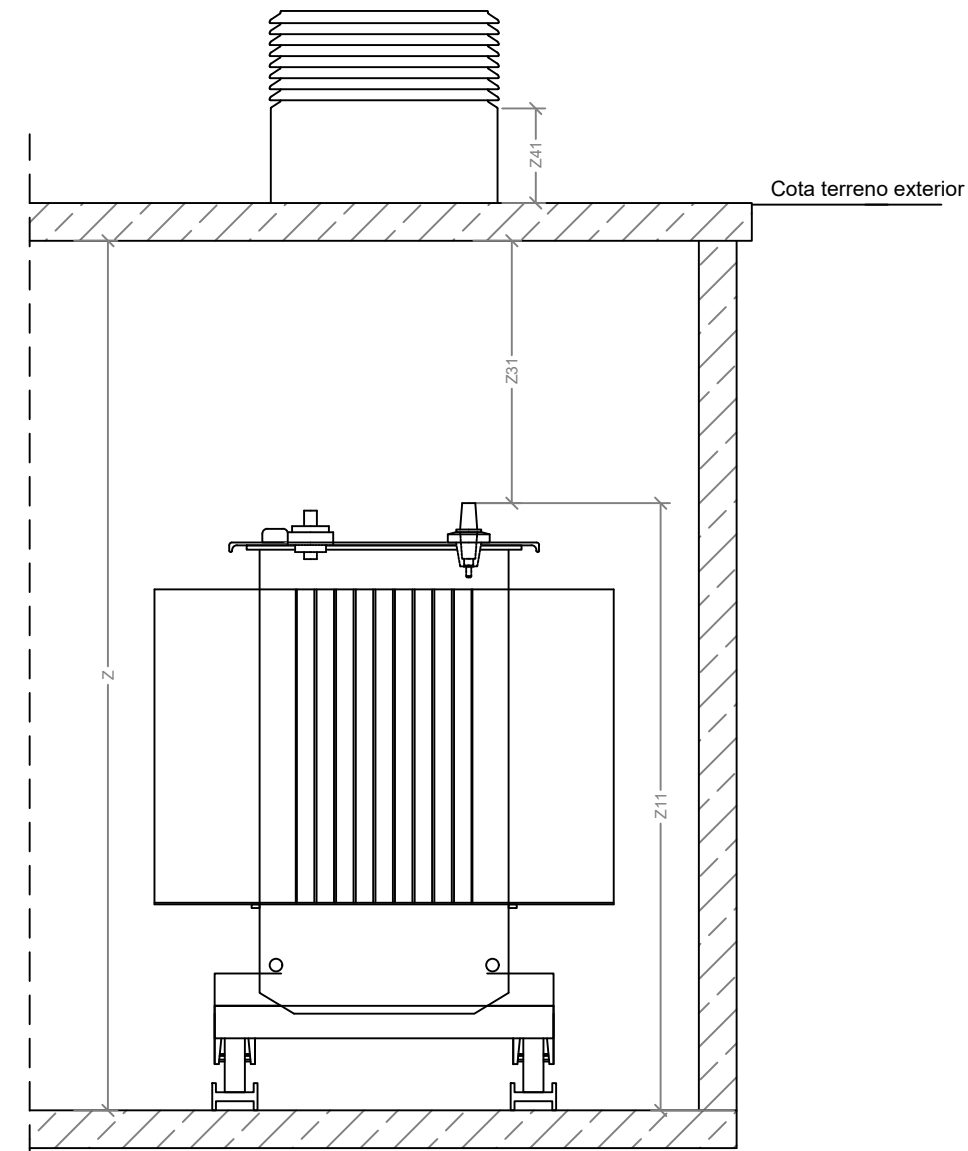
SECCION A-A'
