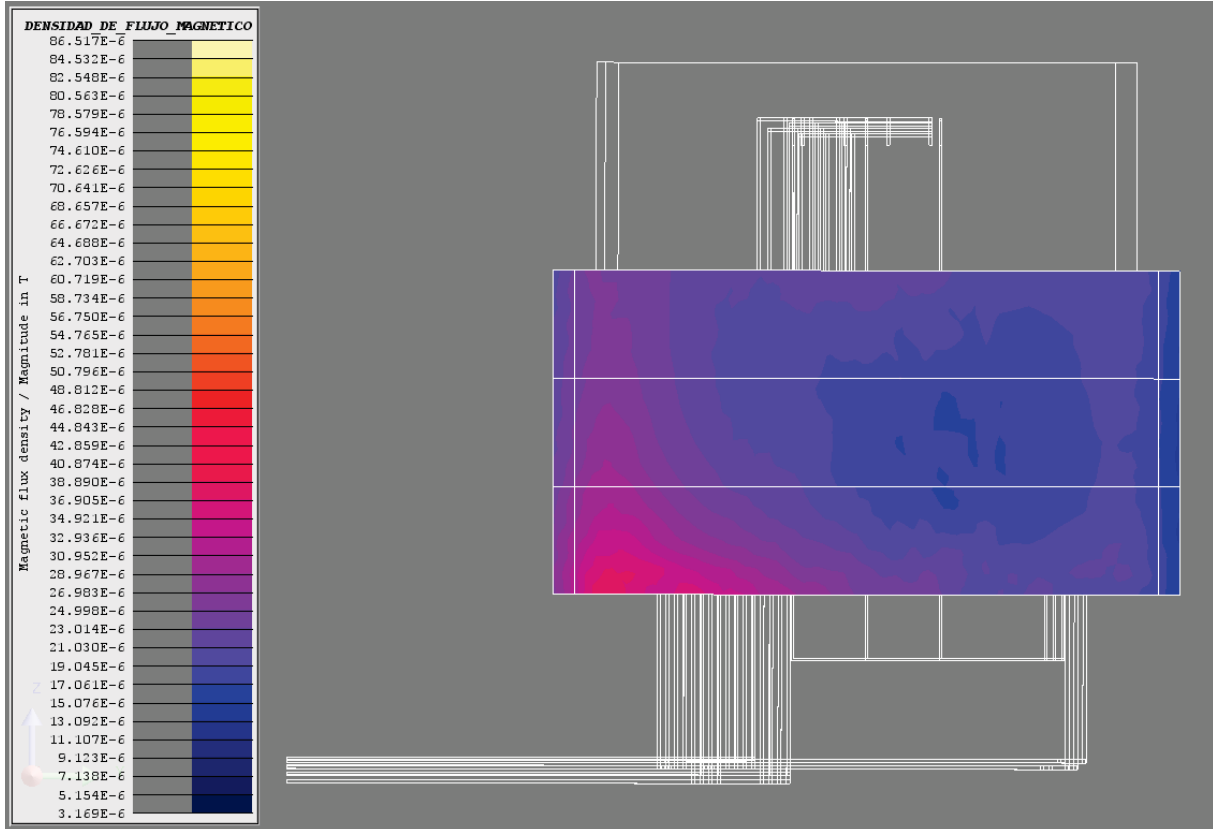
Figura 6. Densidad de flujo magnético (B[T] = Magnitud B) en el panel derecho (2L+1T [Sup]).
