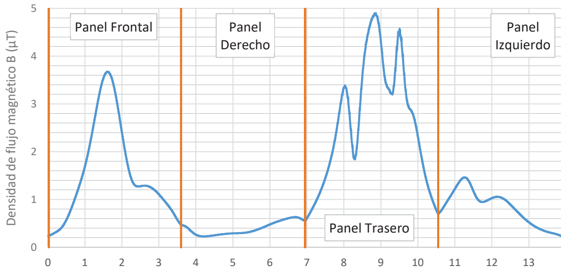
Figura 45. Densidad de flujo magnético ( B[T] = \text{Magnitud } B ) en envolvente situada a 0,5 metros (3L).
