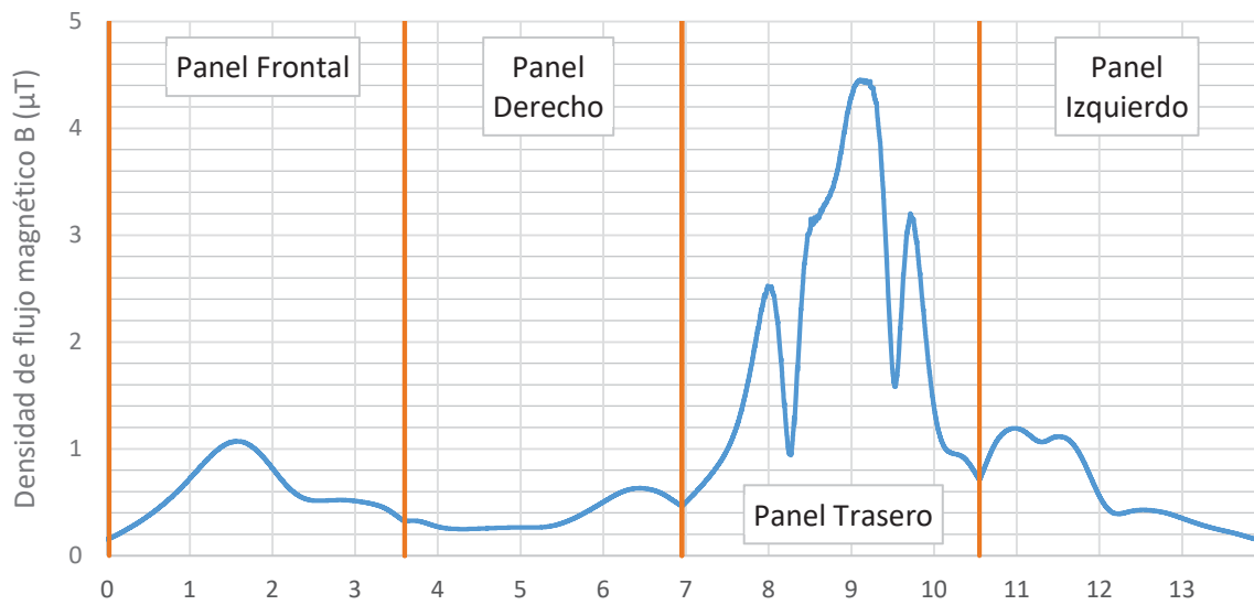
Figura 46. Densidad de flujo magnético ( B[T] = \text{Magnitud } B ) en envolvente situada a 1 metro (3L).
