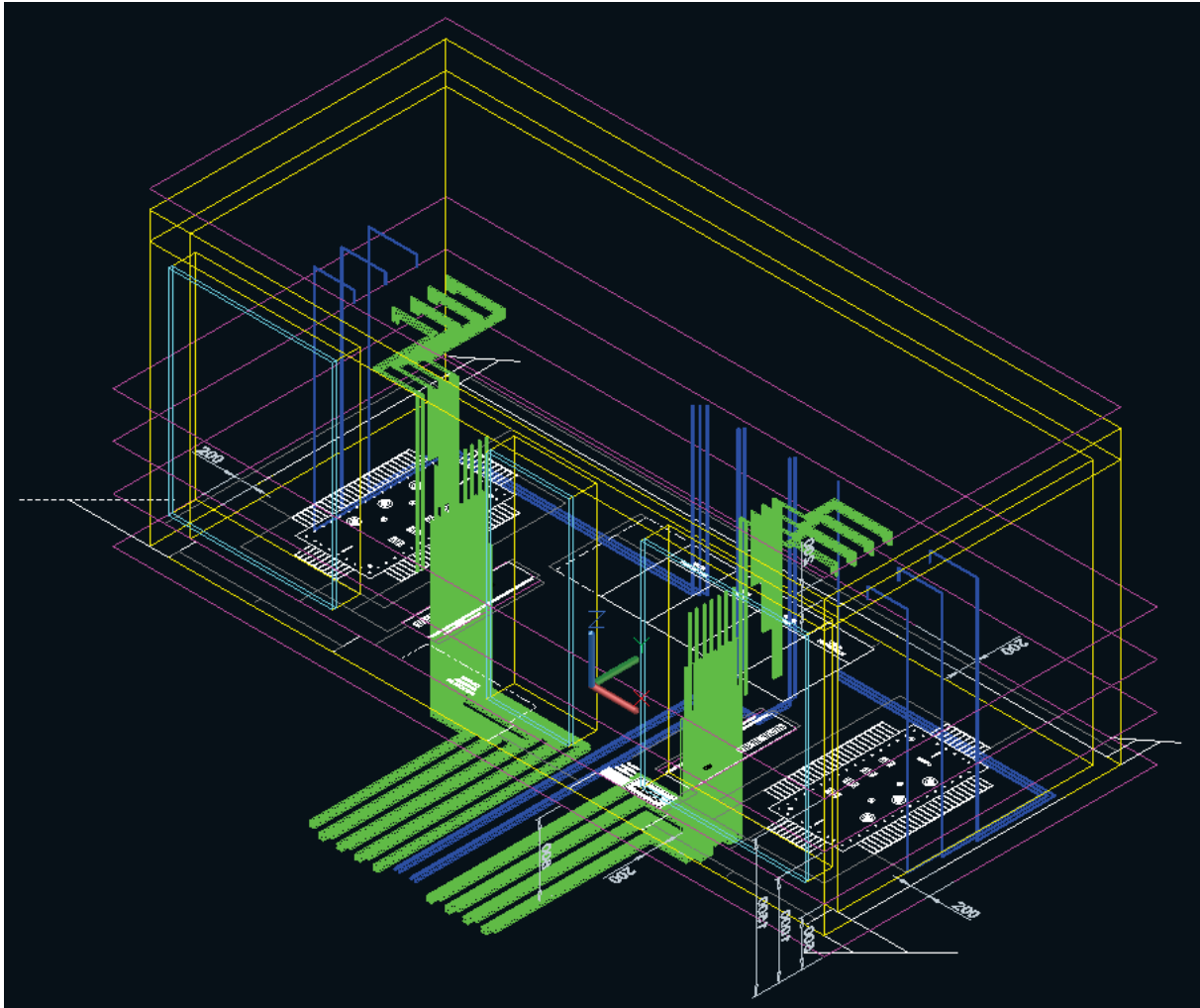
Figura 17. Vista isométrica de la instalación (2L+2T) (cotas en mm).
