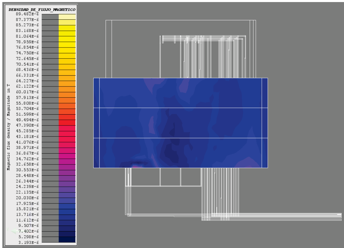
Figura 19. Densidad de flujo magnético ( B[T] = \text{Magnitud } B ) en el panel izquierdo (2L+2T [Sup]).
