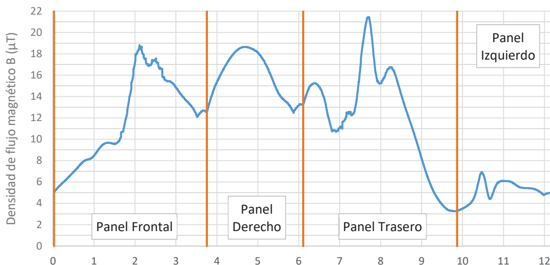
Figura 51. Densidad de flujo magnético ( B[T] = \text{Magnitud } B ) en envoltura situada a 0,5 metros (2L+1T [Semi]).
