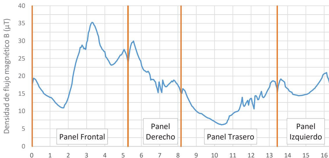
Figura 9. Densidad de flujo magnético (B[T] = Magnitud B) en envolvente situada a 0,5 metros (2L+1T [Sup]).
