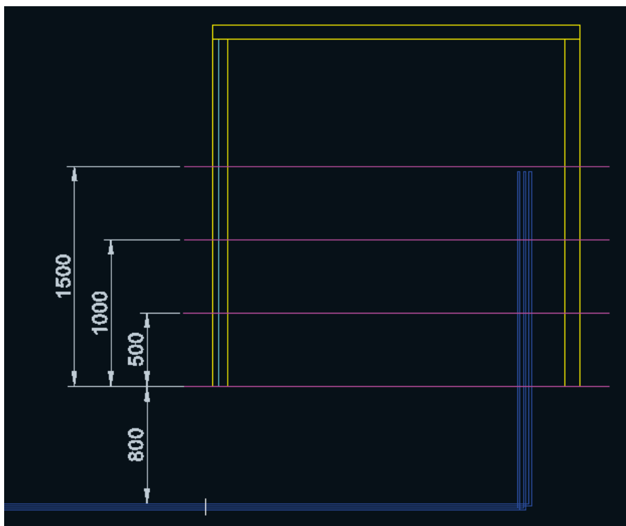
Figura 69. Vista en perfil de la instalación (3L [Sup]) (cotas en mm).
