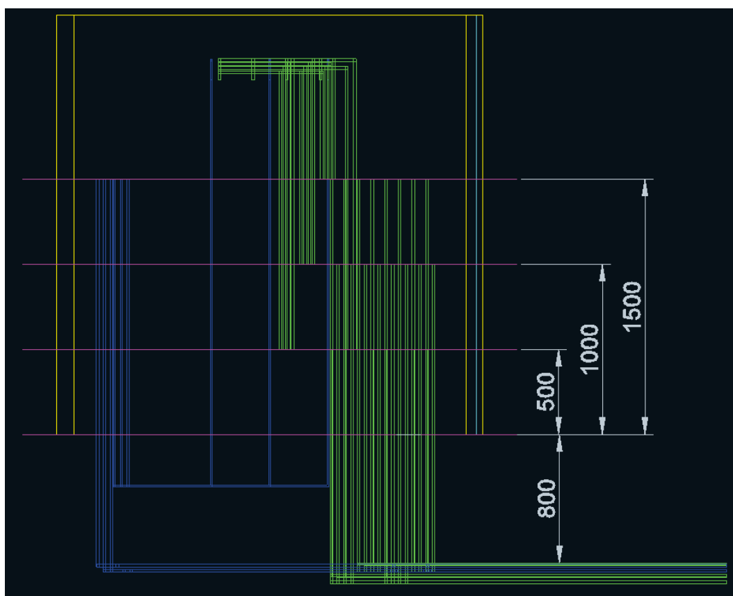
Figura 3. Vista en perfil de la instalación (2L+1T [Sup]) (cotas en mm).
