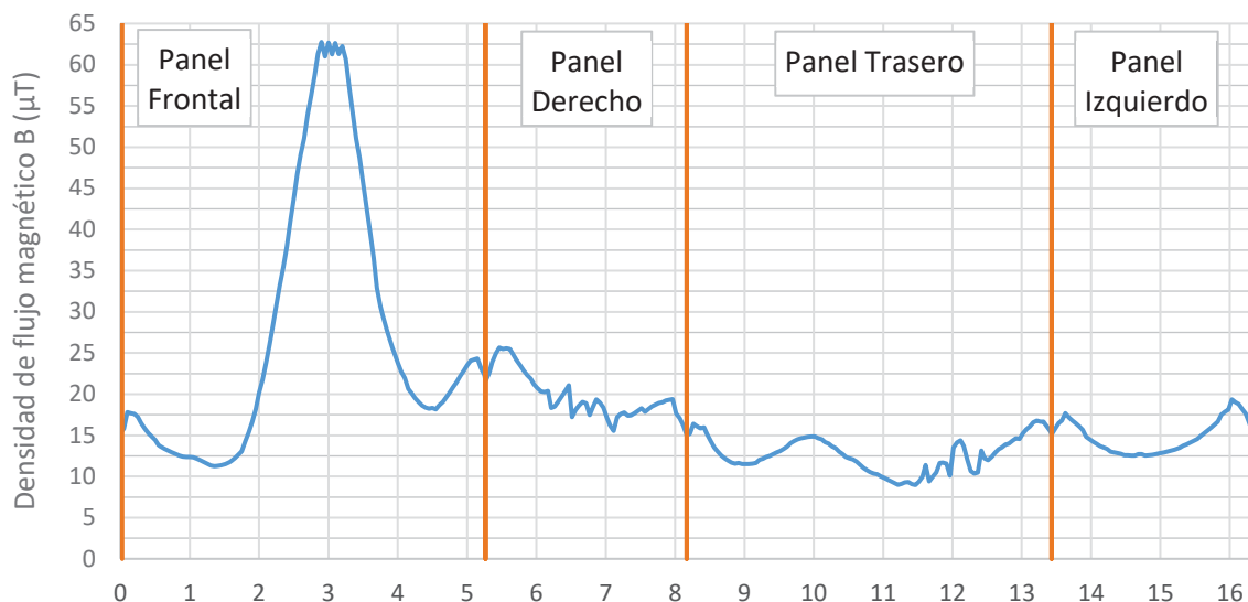
Figura 10. Densidad de flujo magnético (B[T] = Magnitud B) en envolvente situada a 1 metro (2L+1T [Sup]).
