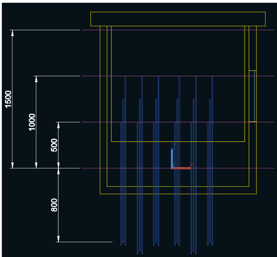
Figura 79. Vista frontal de la instalación (3L [Semi]) (cotas en mm).
