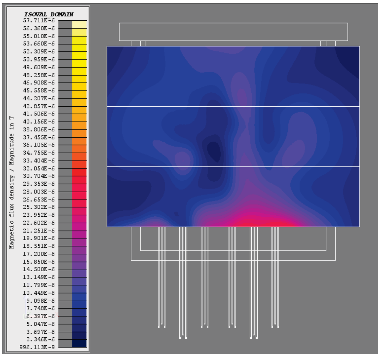
Figura 83. Densidad de flujo magnético ( B[T] = \text{Magnitud } B ) en el panel frontal (3L [Semi]).
