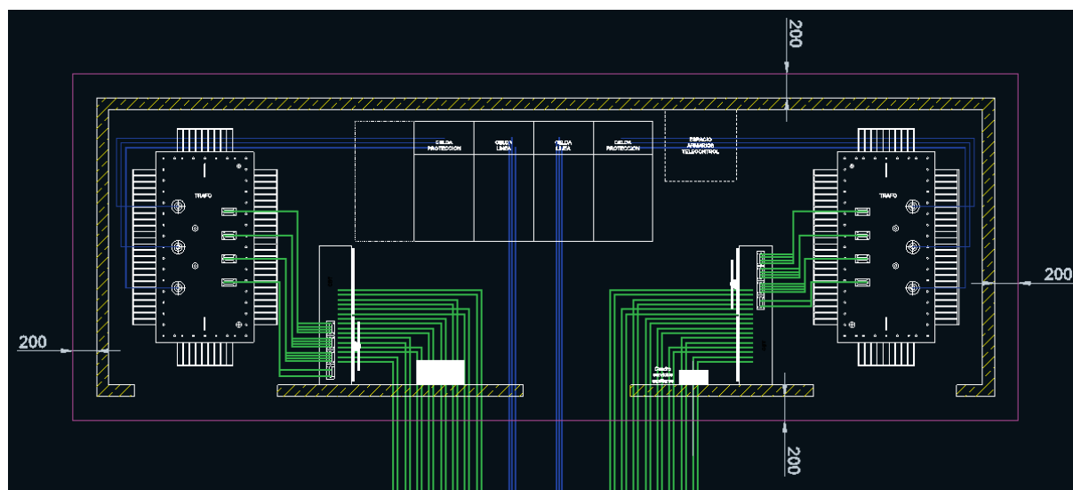
Figura 13. Vista en planta de la instalación (2L+2T [Sup]) (cotas en mm).
