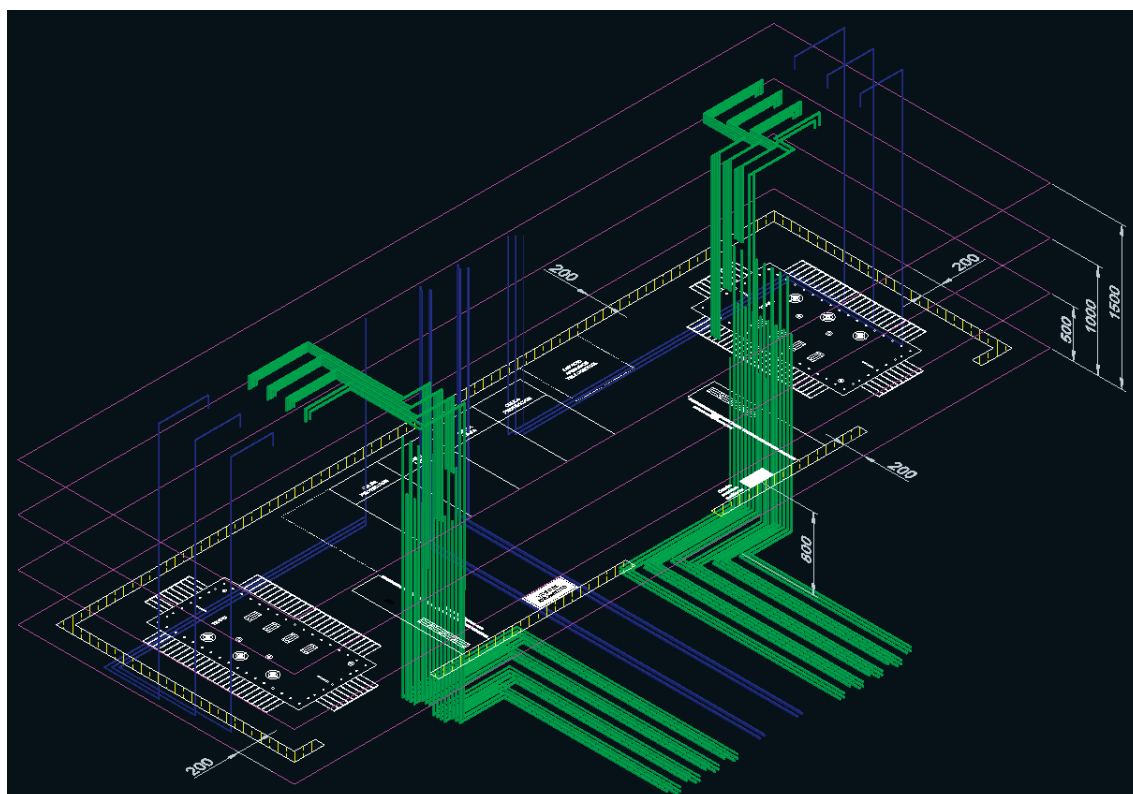
Figura 12. Vista isométrica de la instalación (2L+2T [Sup]) (cotas en mm).
