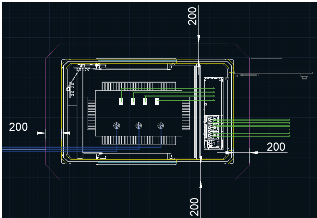
Figura 56. Vista en planta de la instalación (1T [Rural]) (cotas en mm).
