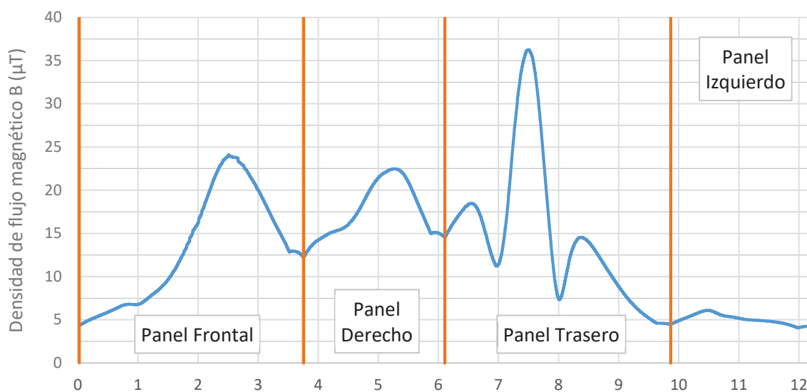
Figura 52. Densidad de flujo magnético ( B[T] = \text{Magnitud } B ) en envoltura situada a 1 metro (2L+1T [Semi]).
