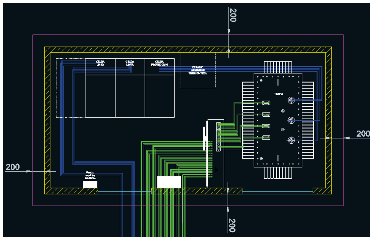
Figura 2. Vista en planta de la instalación (2L+1T [Sup]) (cotas en mm).
